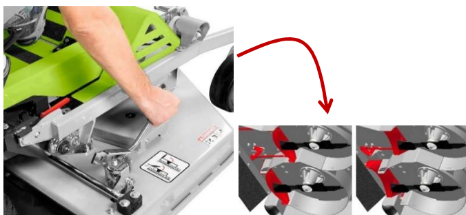
Quick Shift systeem voor makkelijk schakelen tussen mulching en achteruitworp
