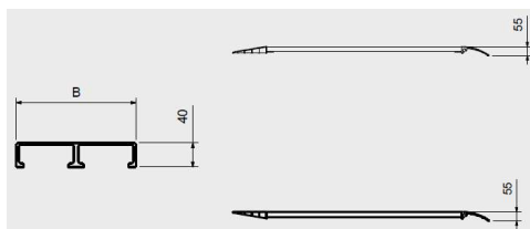
Modèle avec partie finale C040 (sur demande)
