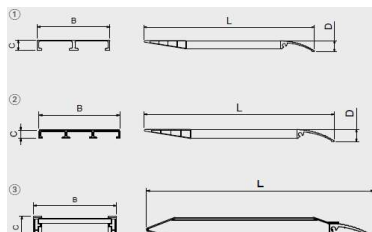
1. Modèle B2 2. Modèle B3 3. Modèle M080
